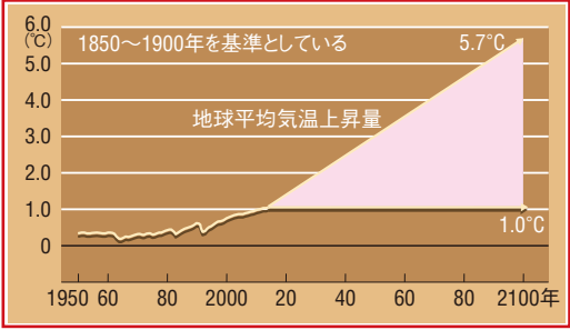
②気温上昇の予測 (IPCC第六次評価報告書)
