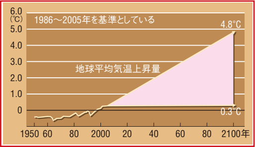
②気温上昇の予測 (IPCC第五次評価報告書)
