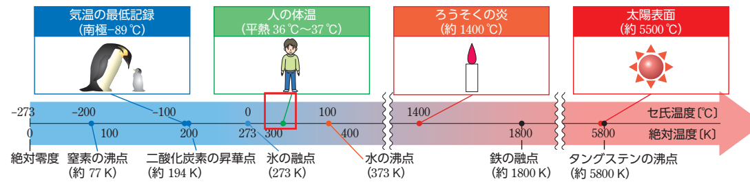
▲ 図3 いろいろな温度 (出典) 理科年表, 『改訂5版化学便覧』
