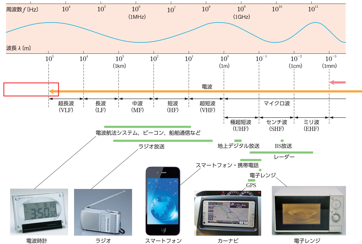
▲ 図1 電磁波の分類 (出典) 総務省, 理科年表 紫外線, X線, γ線の区別は発生のかたによるため, 波長で厳密に分類することはできない。
